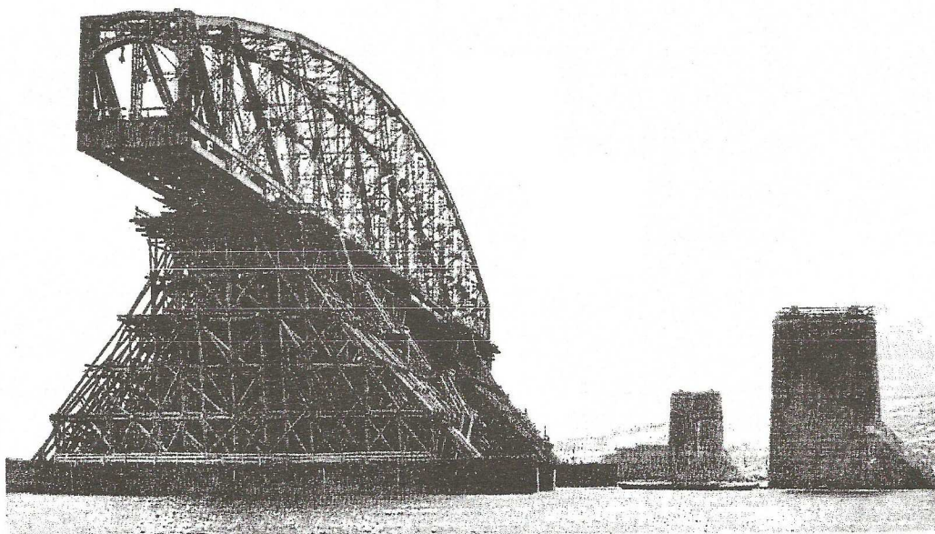
Строительство моста через Волгу под Симбирском. Фото 1915 г.
