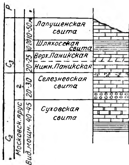
Рис. 20. Разрез карбона Донского купола (по С. В. Семихатовой).
