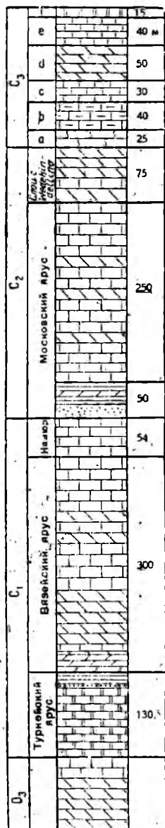
Рис. 17. Разрез карбона Самарской Луки.
