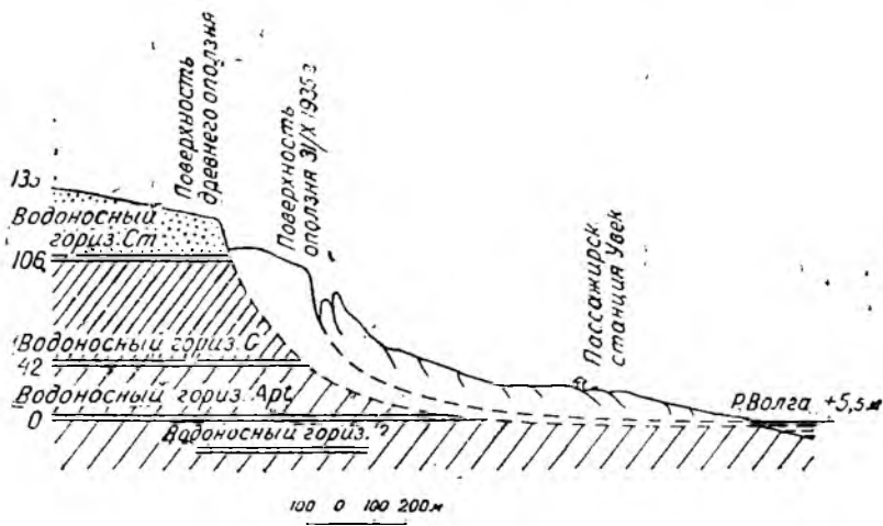
Рис. 51. Геологический профиль горы Увек у Саратова (по Ф. П. Саваренскому).
