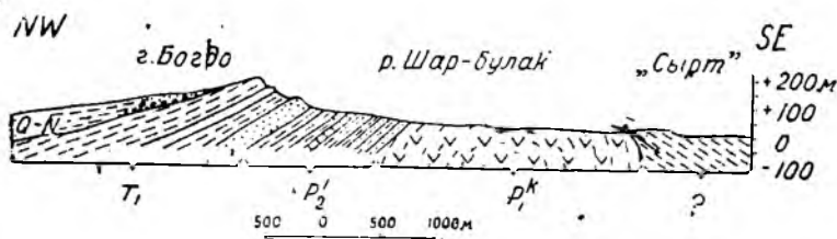
Рис. 71. Разрез через гору Большое Богдо (по А. А. Богданову).
