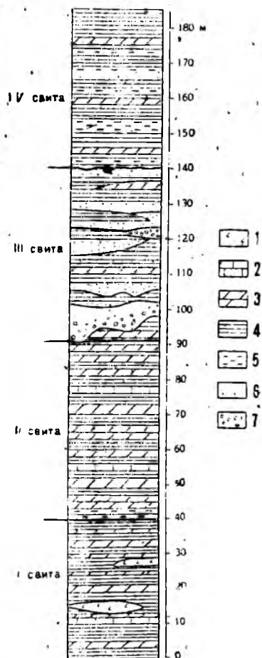
Рис. 23. Схема строения татарских слоев правого берега Волги. 1 — гипс; 2 — доломиты и известняки; 3 — мергеля; 4 — глины; 5 — песчаные глины; 6 — пески и песчаники; 7 — галечники и конгломераты.
