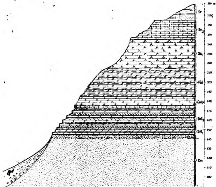
Рис. 50. Геологический разрез Лысой горы у Саратова.
