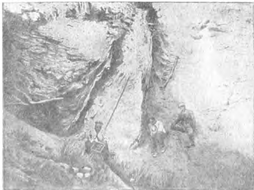
Рис. 58. Сброс в овраге Белевском близ г. Камышина.
