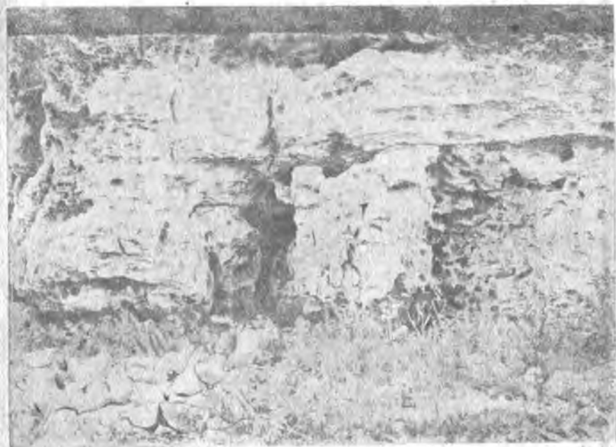
Рис. 45. Обнажение закарстованных известняково-доломитовых пород в Жигулях. (Фото А. А. Баркова).
