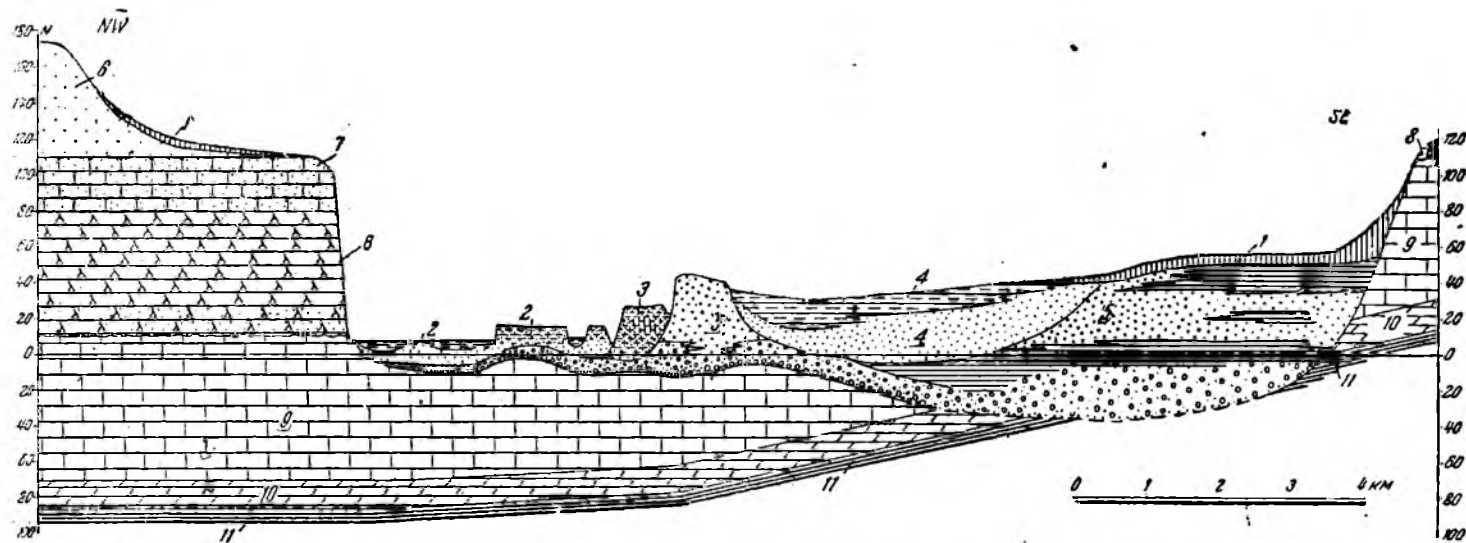
Рис. 66. Схематический разрез долины Волги в районе с. Белогродни и Витман. (Строение террас долины Волги дано в интерпретации Н. И. Николаева.)
