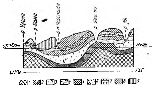
Рис. 9. Разрез Вятско-Улеминского вала, Лаишевского прогиба и Сокско-Шешминского вала (по Е. И. Тихвинской).
