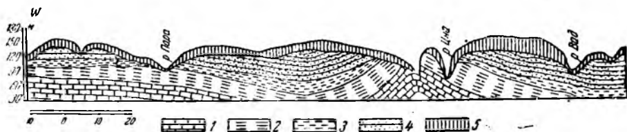
Рис. 7. Разрез через южную часть Окско-Цнинского вала (по Н. А. Богословскому).
