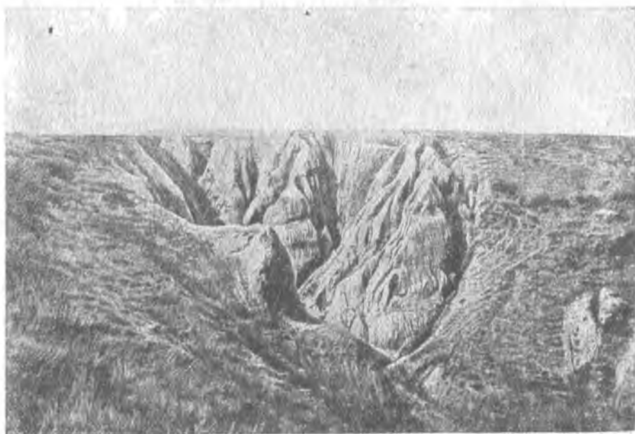
Рис. 62. Обнажение толщ красных суглинков Александровского грабена: (Фото А. П. Павлова).
