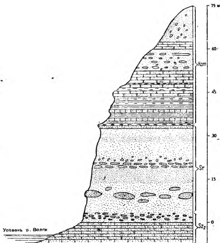
Рис. 63. Разрез правого берега Волги у с. Пролейки. Sz 2 — верхнесызранские слои; Sr — саратовские слои; Кам — камышинские слои.
