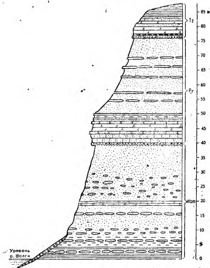
Рис. 64. Геологический разрез правого берега Волги у с. Широкого.
