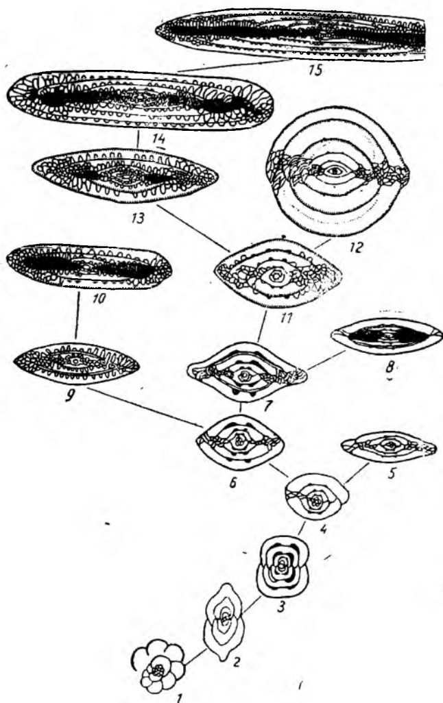
Рис. 18. Схема филогенетического развития сем. Fusulinidae (по Д. М. Раузер-Черноусовой и А. В. Фурсенко).
