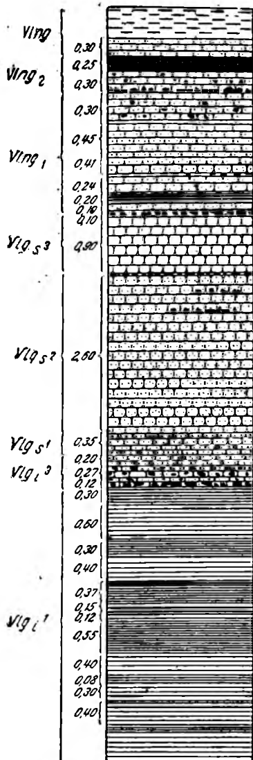
Рис. 47. Геологический разрез валанжинских и волжских слоев у с. Кашпир (пс Е. В. Орловой).
