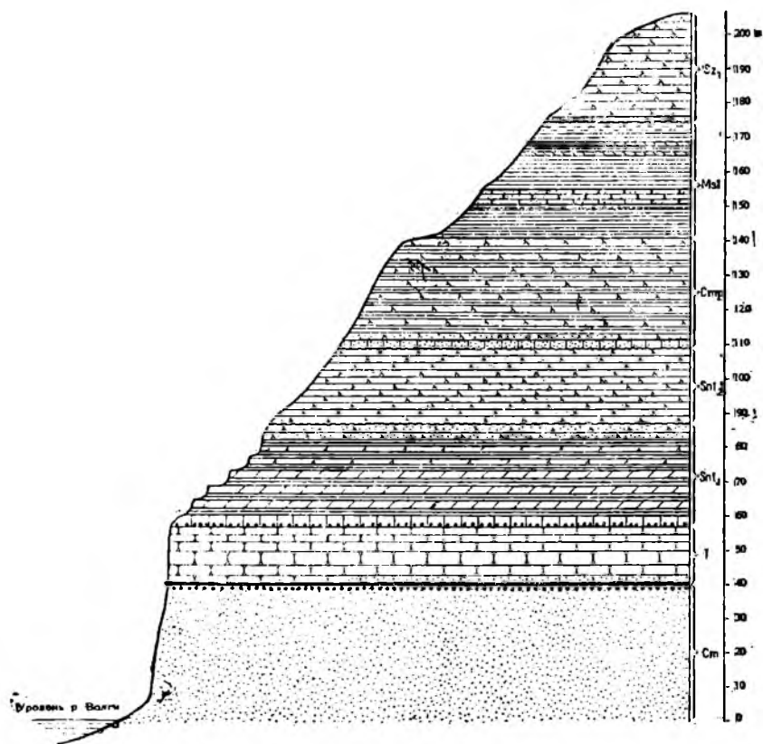
Рис. 54. Геологический разрез горы Сырт у Банников.
