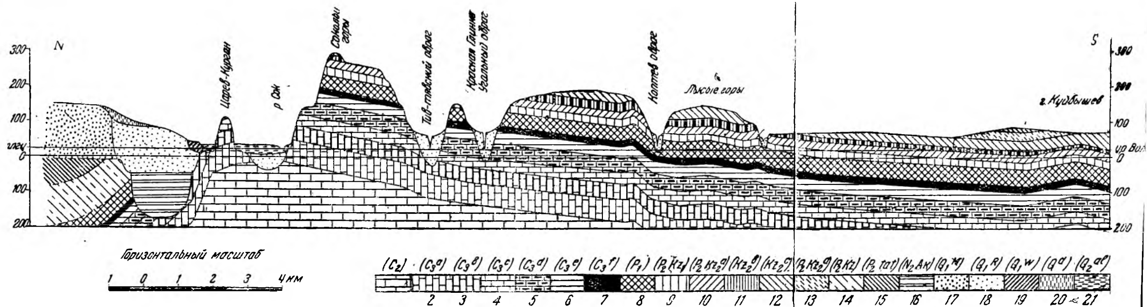
Рис. 43. Геологический профиль по левому берегу Волги от района Царева Кургана до г. Куйбышева.
