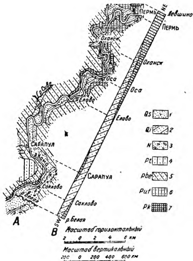
Рис. 76. А — схематическая геологическая карта долины р. Камы от г. Перми до устья р. Белой. Б — схема условий залегания пермских образований вдоль долины р. Камы от г. Перми до устья р. Белой (по Б. В. Селивановскому и Е. Н. Ларьоновой).
