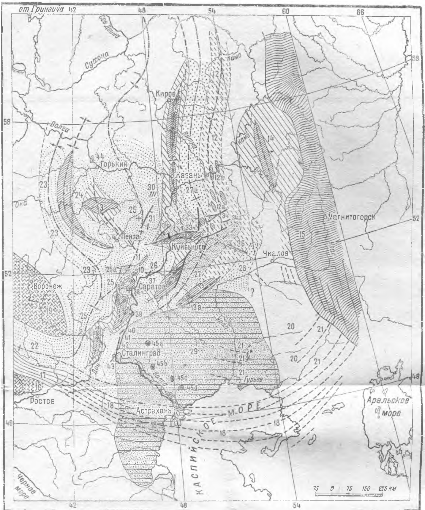
Рис. 6. Схематическая тектоническая карта Поволжья (Составил Е. В. Милановский).
