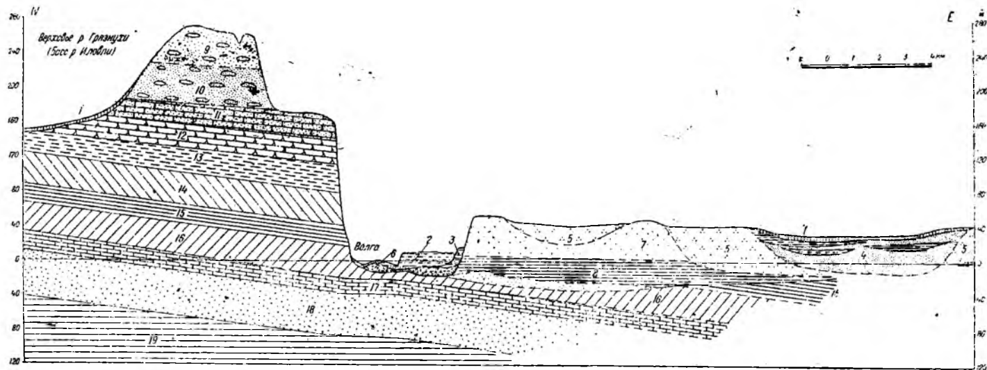
Рис. 67. Схематический геологический профиль долины Волги в районе с. Миллер и Белокаменки. (Составлен по данным бурения Нижневолгостроя, данным профиля Н. И. Николаева и материалам автора.)
