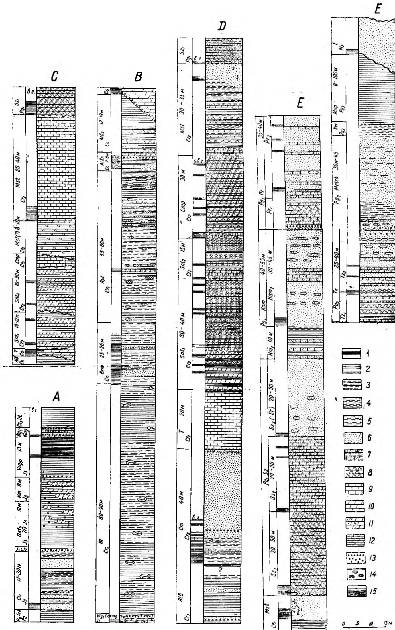
Рис. 24. Стратиграфические колонки мезозойских и палеогеновых отложений правобережья Волги.
