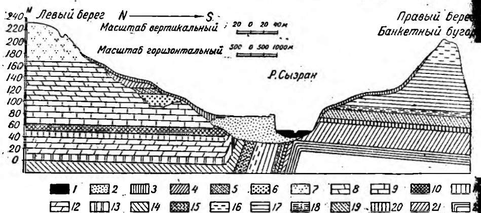
Рис. 46. Разрез через долину р. Сызрана в районе с. Репьевки.
