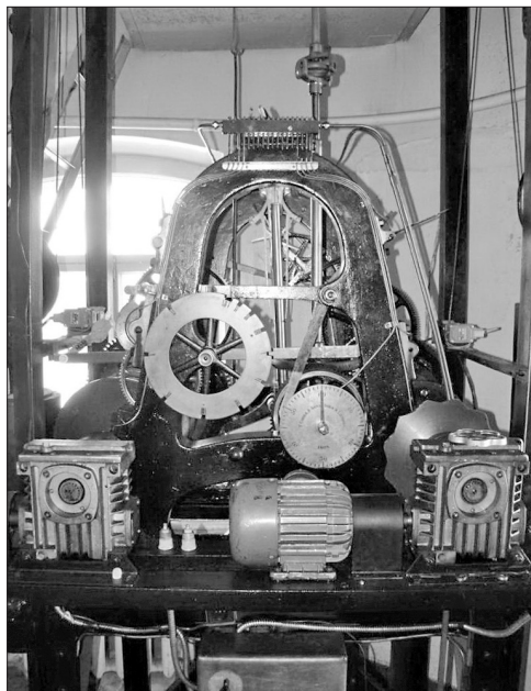
Часовой механизм компании T. Cooke & Sons. York & London. Музей одного экспоната «Симбирские городские часы». Источ.: Фонды «Историко-мемориального центра-музея И. А. Гончарова»
