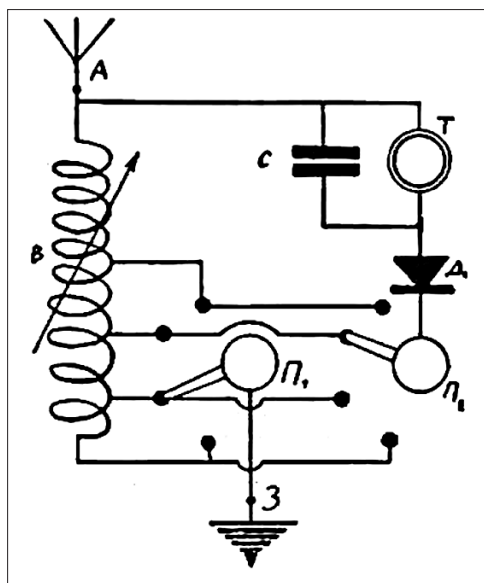
Общая схема приёмника системы инж. Шапошникова. Источ. Наука и техника. – 1928. – № 36 (сент.). – С. 12–14
