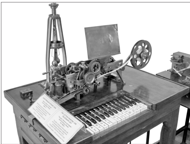
Буквопечатающий телеграфный аппарат Юза с гиревым приводом. Производство фирмы «Сименс и Гальске», г. Санкт-Петербург, 1870-е – 1880-е гг.
