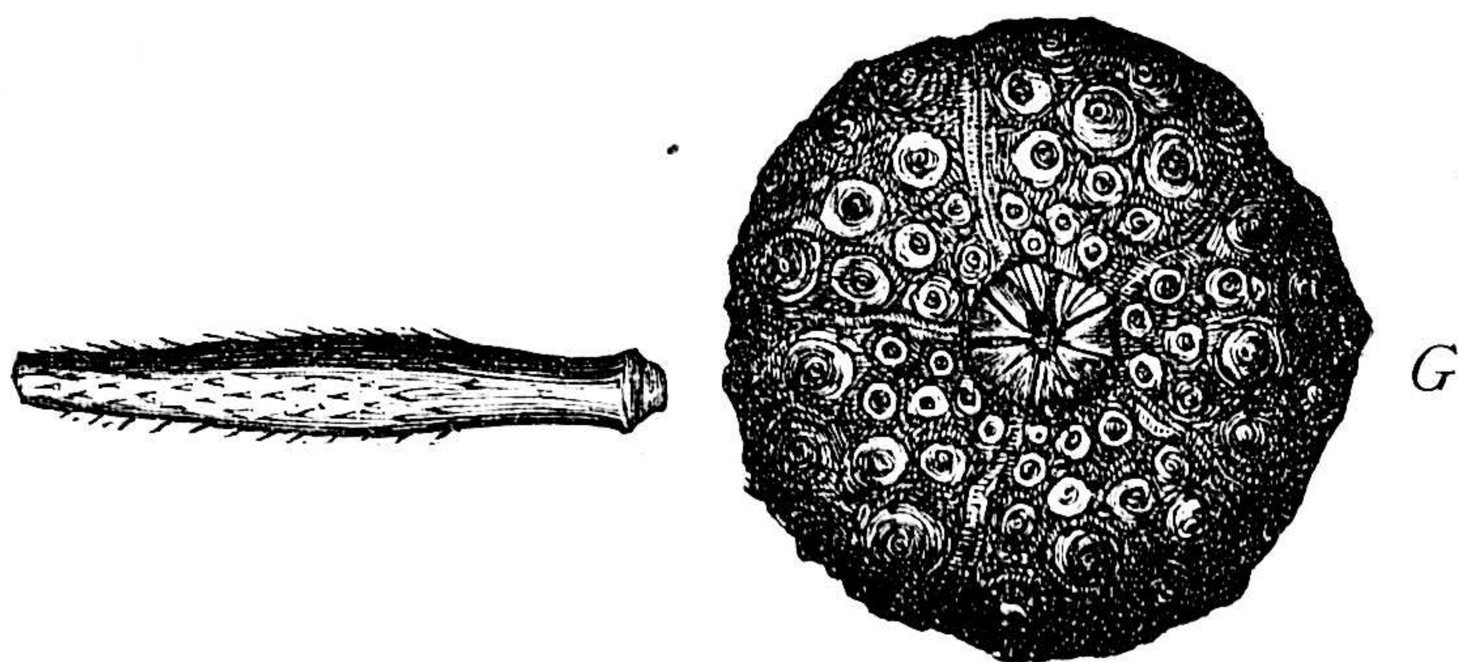
Archæocidaris rossicus . (Слѣва представлена одна изъ его иголь).
