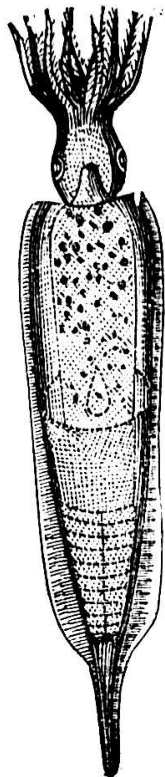
Идеальное изображеніе животнаго вымершихъ белемнитовъ.
